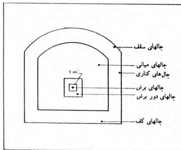
شکل ۶-۷ چال‌های مختلف در یک جبهه کار
