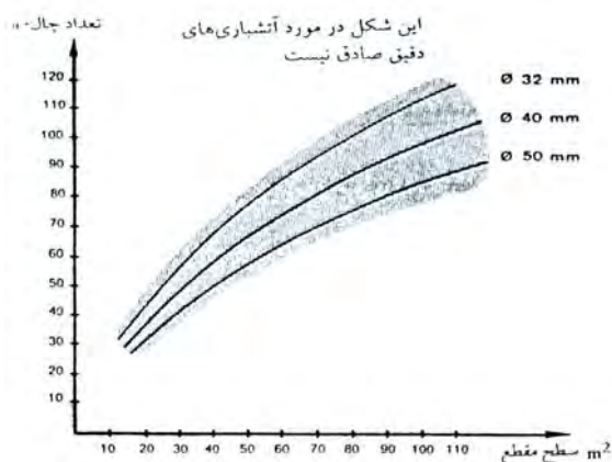
شکل ۶-۴- تعداد چال‌های لازم برای تونل‌های با مقاطع مختلف
