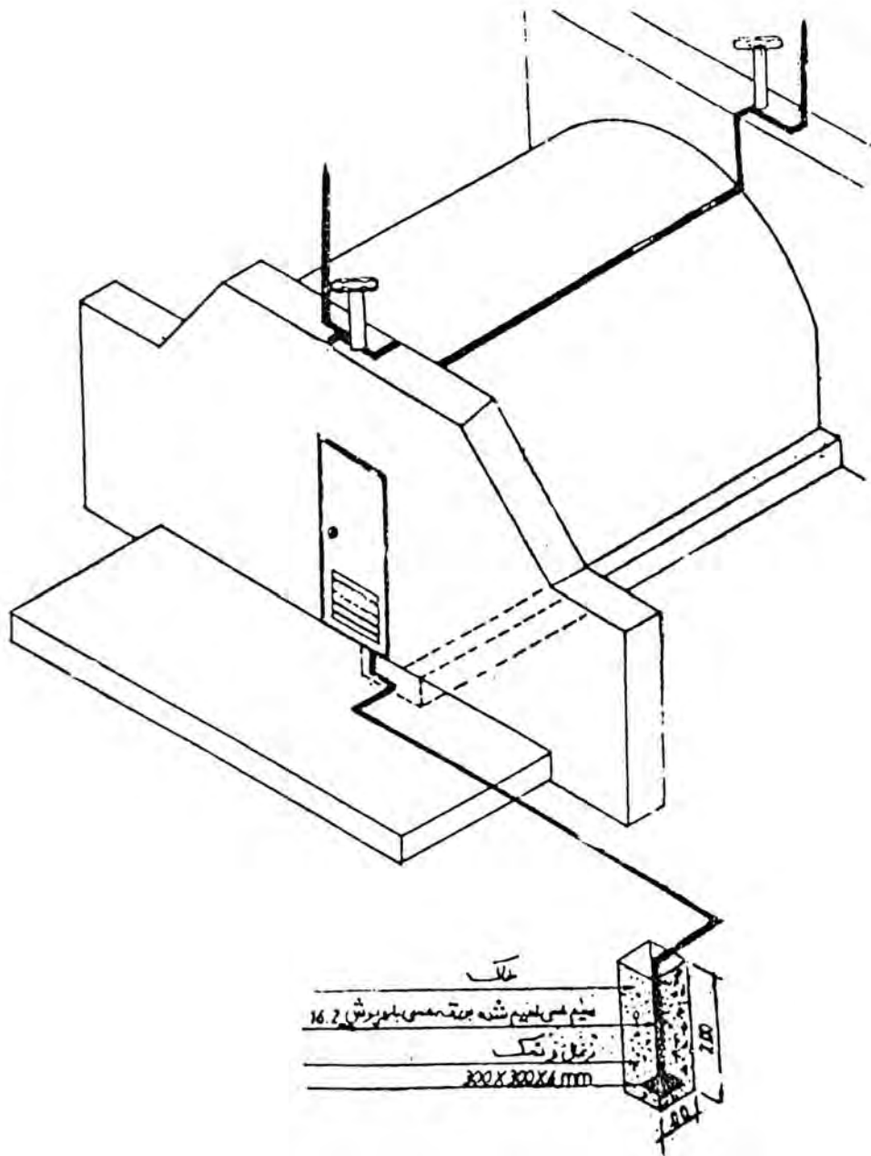
شکل ۴-۶- سیستم برق گیر و اتصال زمین
