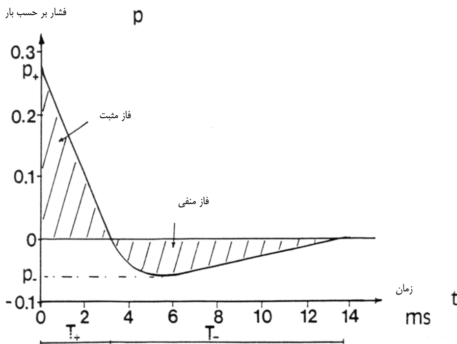
شکل ۶-۱۱- موج ضربه و تغییرات آن نسبت به زمان در فاصله ۵ متری از انفجار آزاد ۱ کیلوگرم T.N.T
