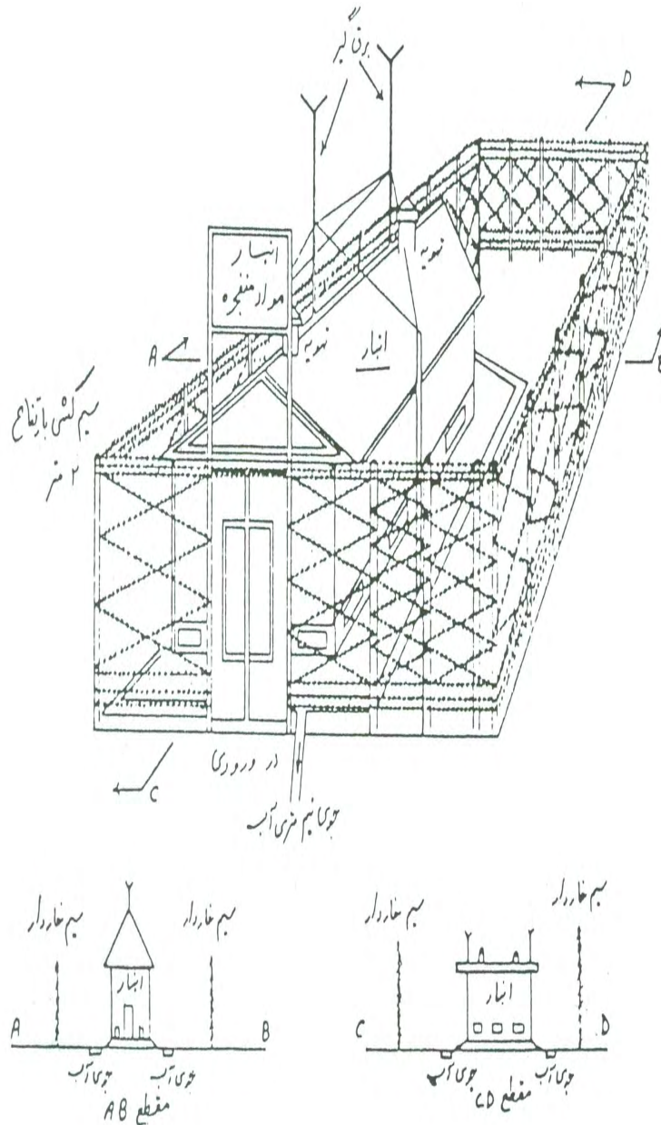
شکل ۴-۷- نقشه اجرایی یک انبار مواد ناریه
