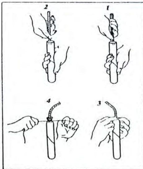
شکل ۵-۲- مراحل مختلف چاشنی گذاری
