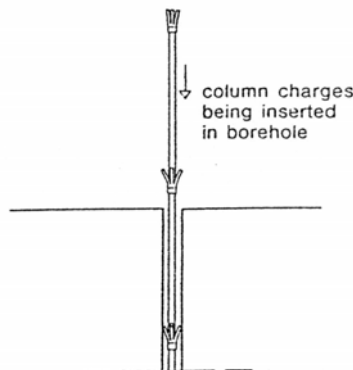
شکل ۷-۲- خرج گذاری لولهای مواد منفجره همراه با پره های پلاستیکی برای جلوگیری از تماس خرج با دیواره چال
