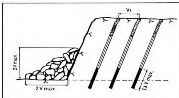
شکل ۶-۱- نحوه آتشیاری در معادن سطحی
