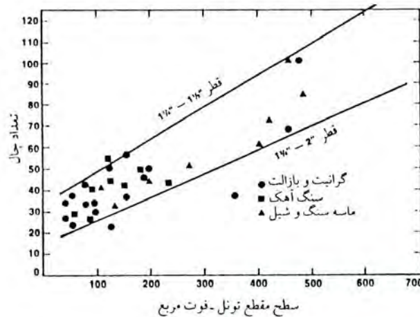
شکل ۶-۵- تعداد چال‌های لازم برای تونل‌های با مقاطع مختلف
