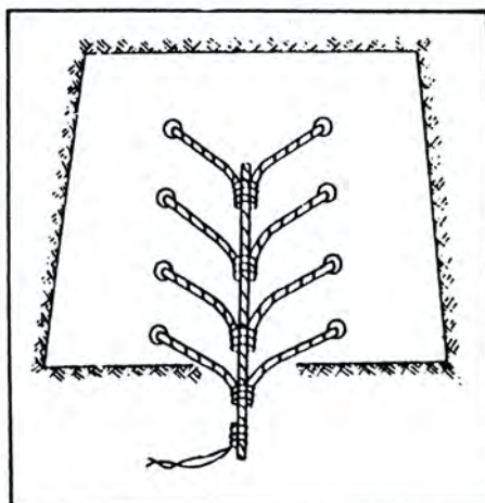
شکل ۵-۸- اتصال فتیله چال‌ها به حالت سری- موازی
