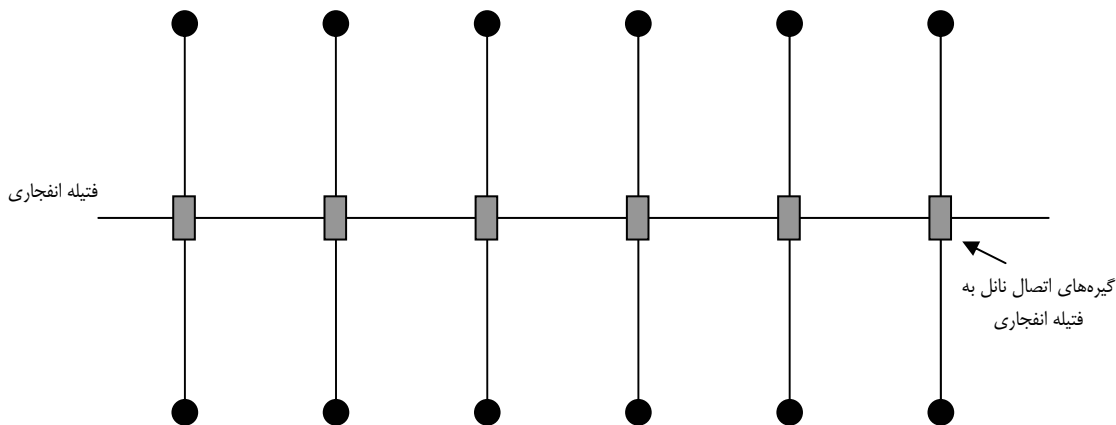
شکل ۵-۱۱- نحوه استفاده از سیستم ترکیبی نائل و فتیله انفجاری
