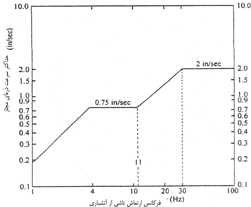
شکل ۶-۱- تغییرات اوج سرعت ذره‌ای مجاز نسبت به فرکانس ارتعاش
