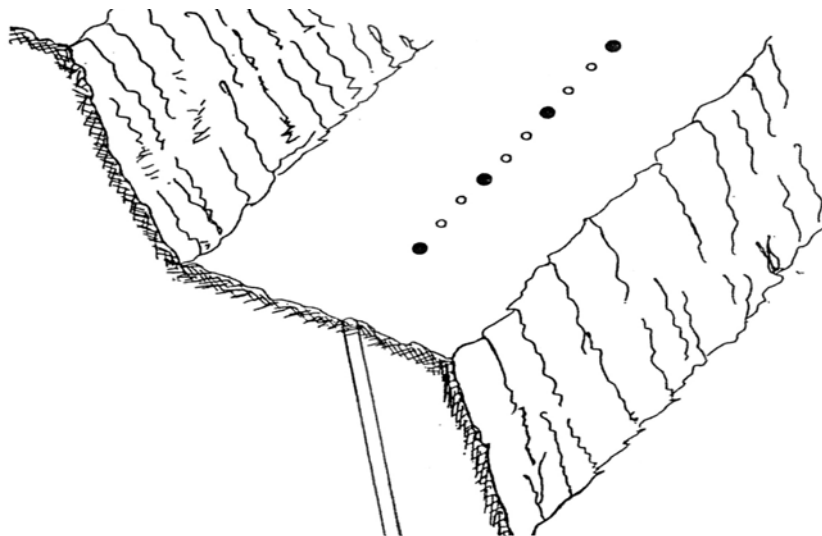
شکل ۷-۵- ترکیب روش آتشباری بالشی با چال خالی
