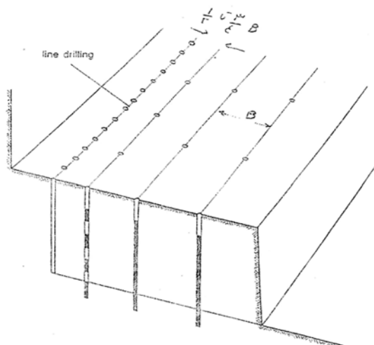
شکل ۷-۷- آرایش و خرج گذاری چال‌ها در آتشیاری با چال خالی
