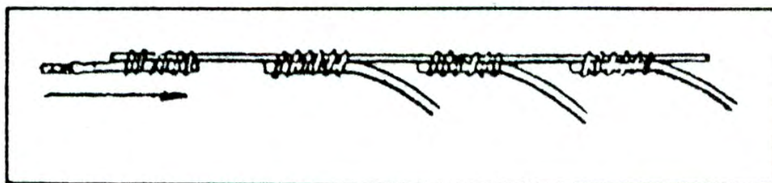
شکل ۵-۷- اتصال فتیله چال‌ها به حالت سری
