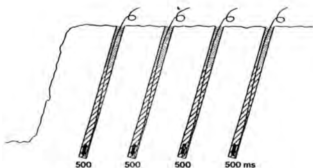
شکل ۵-۹- خرج گذاری سیستم نائل
