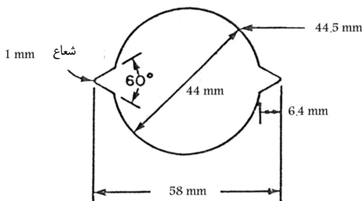
شکل ۷-۸- ابعاد شیاری در چال‌های کنترل شکاف قطر چال ۴۴ میلی‌متر است.
