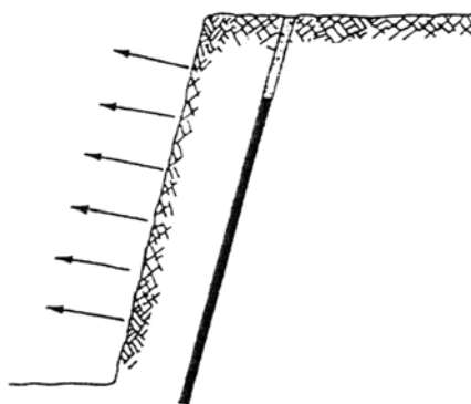
شکل ۶-۱۳- وضعیت ایده‌آل انفجار از نظر پرتاب سنگ
