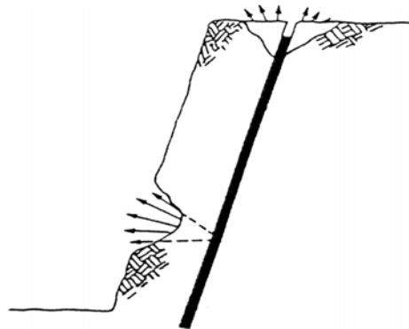
شکل ۶-۱۴- دو وضعیتی که باعث افزایش پرتاب می‌شوند
