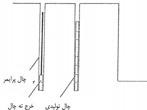
شکل ۷-۳- خرج ته چال در چالهای کناری در آتشباری
