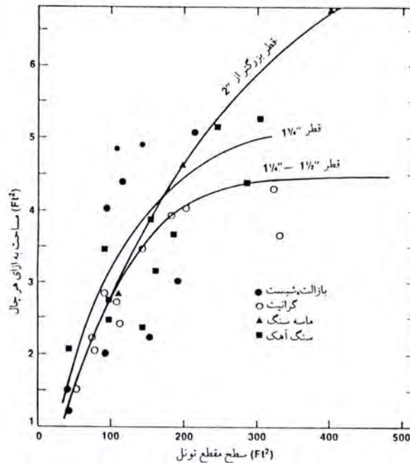
شکل ۶-۶- رابطه بین قطر چال و سطح مقطع تونلها
