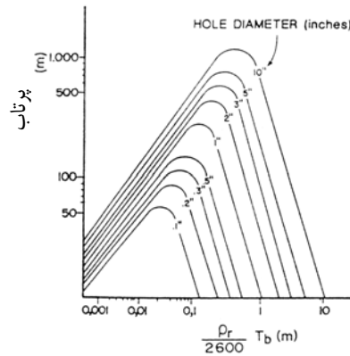
شکل ۶-۱۷- اندازه پرتاب در مقایسه با اندازه قطعات
