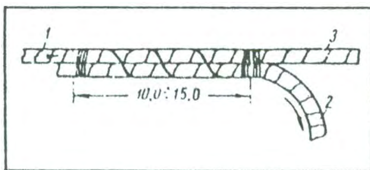
شکل ۵-۶- اتصال فتیله چال‌ها به فتیله اصلی
