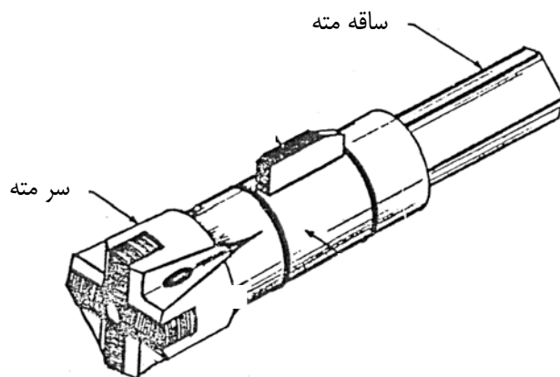
شکل ۷-۹- قطعه شیاردهنده که بر میله حفر چال نصب شده است.
