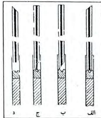
شکل ۵-۱- وضعیت صحیح و غلط فتیله گذاری
