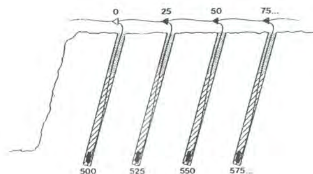
شکل ۵-۱۰- اتصال چال‌ها به حالت سری
