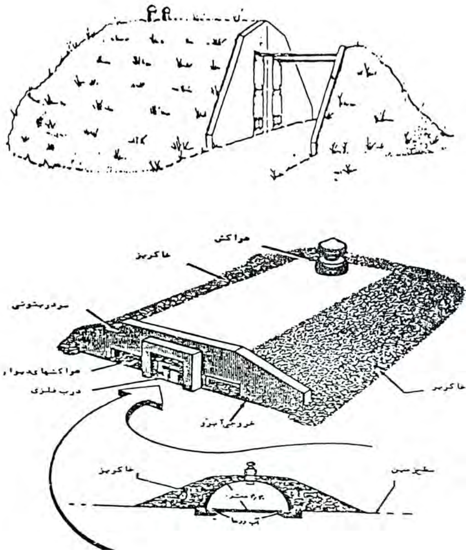
شکل ۴-۱- ساختمان انبار مواد ناریه نوع ایگلو
