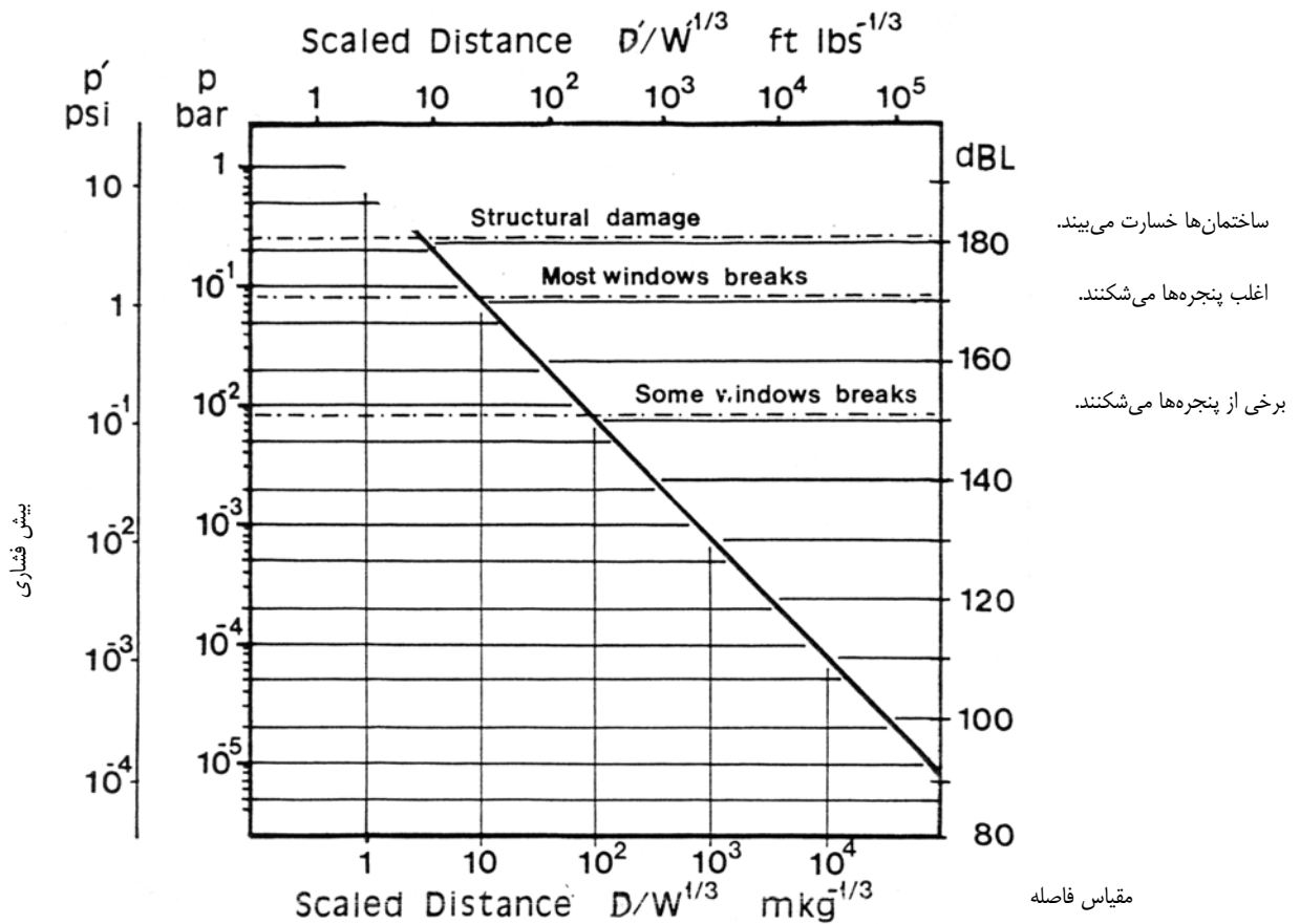
شکل ۶-۱۲- رابطه بین فشار لرزش هوا و فاصله در مقیاس تمام لگاریتمی
