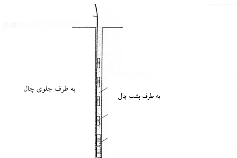
شکل ۷-۴- خرج‌گذاری در آتشباری بالشی
