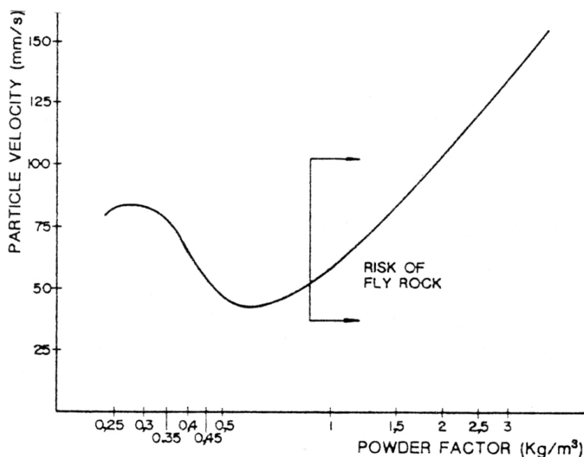
شکل ۶-۸- تاثیر خرج ویژه بر شدت لرزش
